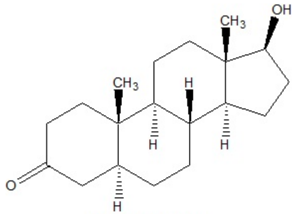
Androstanolone
