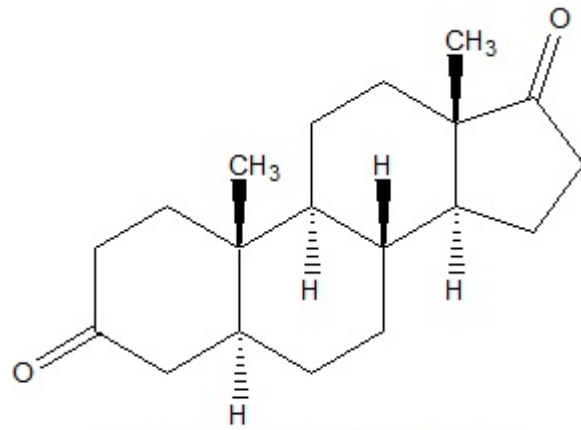
5alpha-Androstan-3,17-dione
